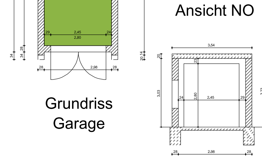
Schnitt
