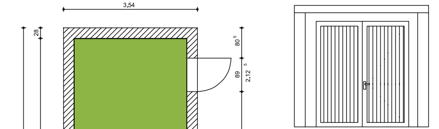
Ansicht SW
